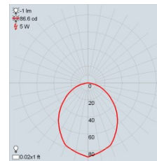
Lentille Blanche Givrée – 300lm/pi – 4000K
